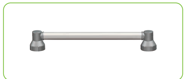
Haltegriff 50 cm , Art.Nr. 61.000040 Gesamtlänge 51,6 cm
